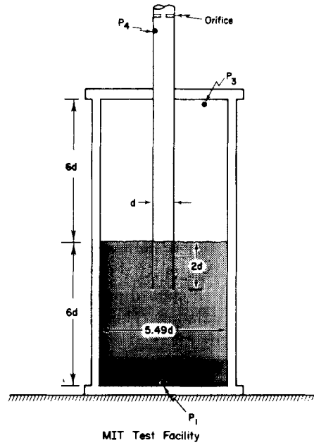
FIG. 12. Schematic of MIT single-vent test apparatus.
